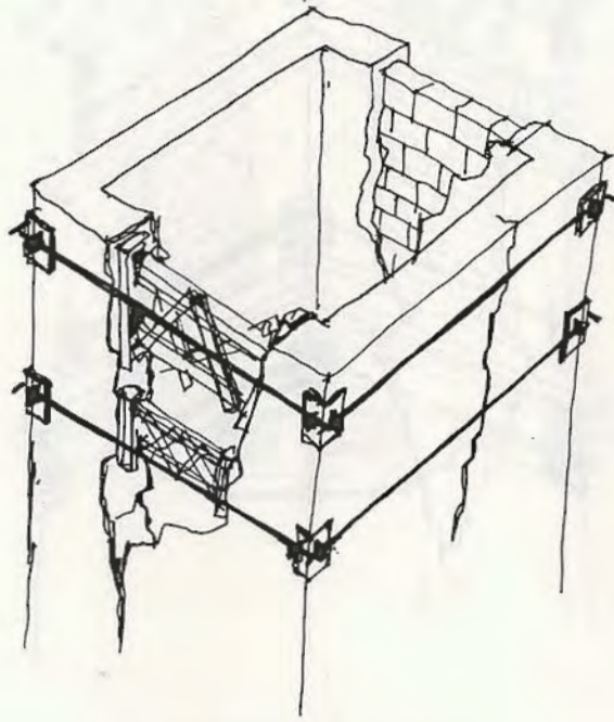
إستعادة الاستمرارية الانشائية
