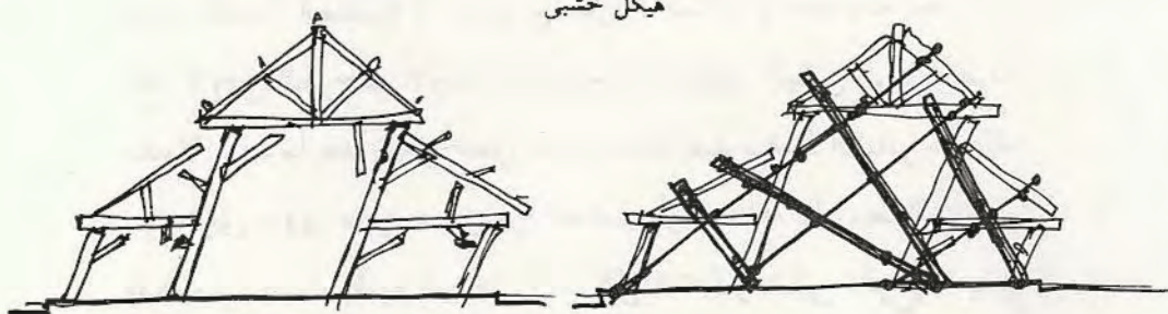
التثبيت المؤقت
