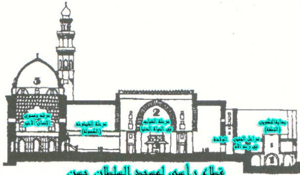
قطاع رأسي لمسجد السلطان حسن مراحل عمر الإنسان من خلال الفراغات
