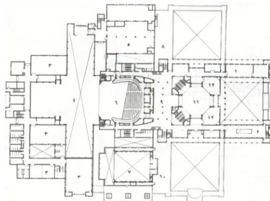
مسقط أفقي للدور الأول
