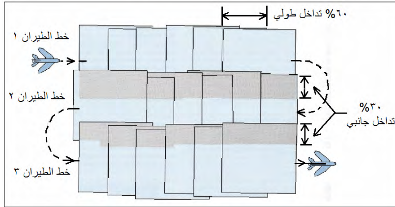
شكل (١٤-٥) التداخل الجانبي
