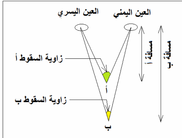
شكل (٦-٥) مفهوم الإبصار المجسم في العين البشرية
