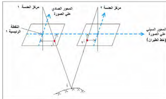
شكل (١٥-٥) الابتعاد علي الصور الجوية
