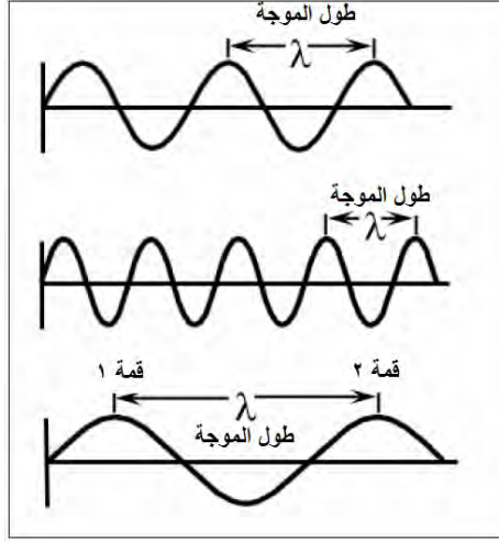
شكل (٢-٣) الطول الموجي للضوء الكهرومغناطيسي
