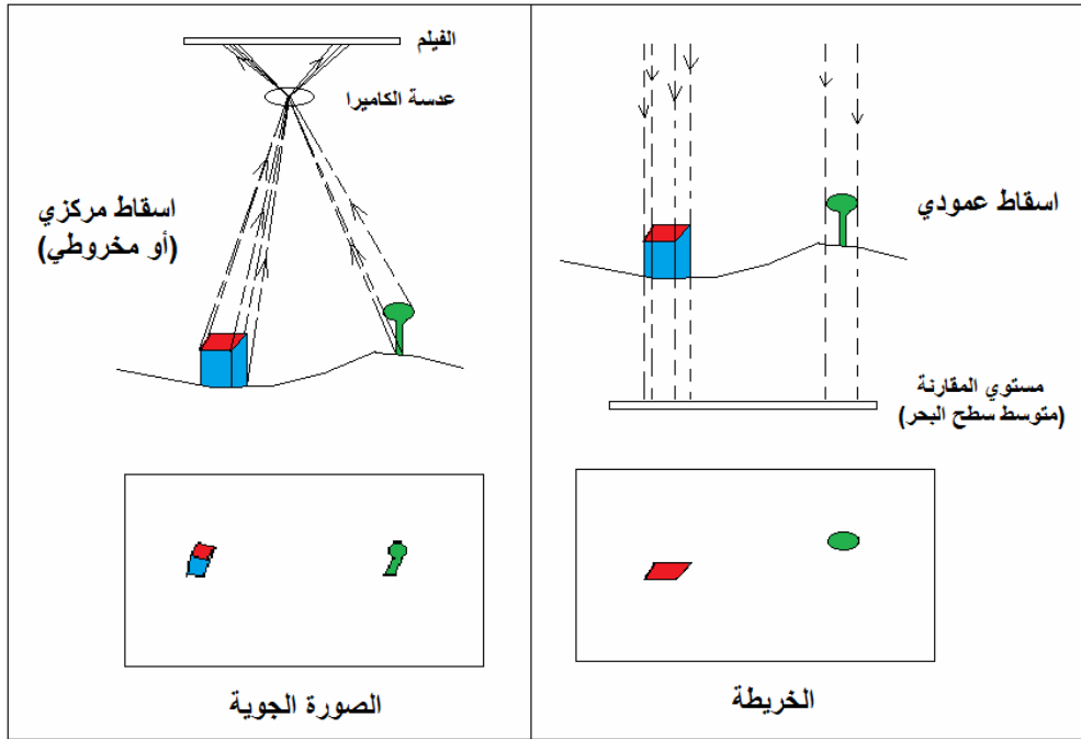
شكل (٢-٩) فرق الإسقاط بين الخريطة والصورة الجوية
