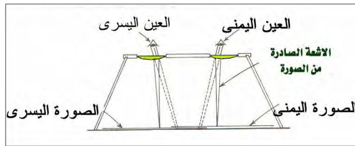
شكل (٨-٥) مفهوم عمل أجهزة الاستريسكوب
