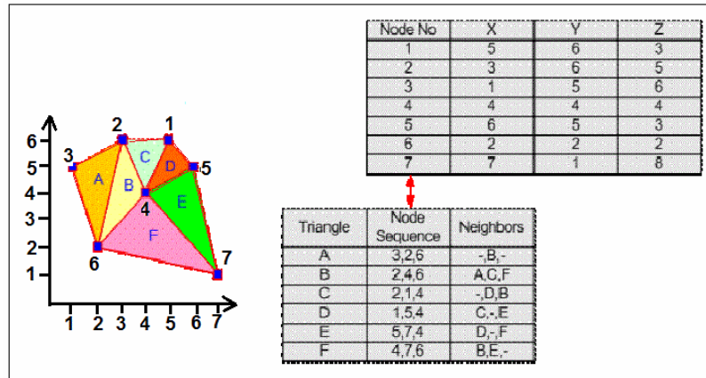
شكل (٨-٥) مثال توضيحي لإنشاء المثلثات غير المنتظمة (نقلا عن عبده ٢٠٠٥)
