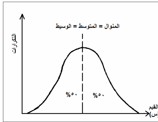
شكل (٢-٢) التوزيع المتماثل
