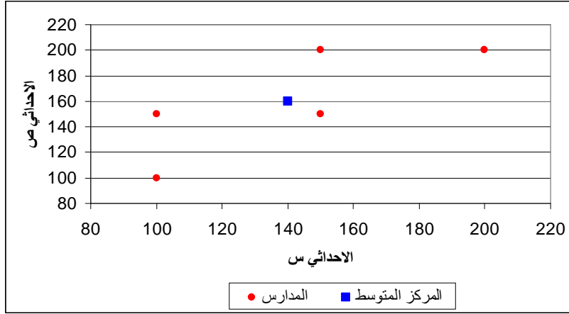
شكل (٣-١) المركز المتوسط
