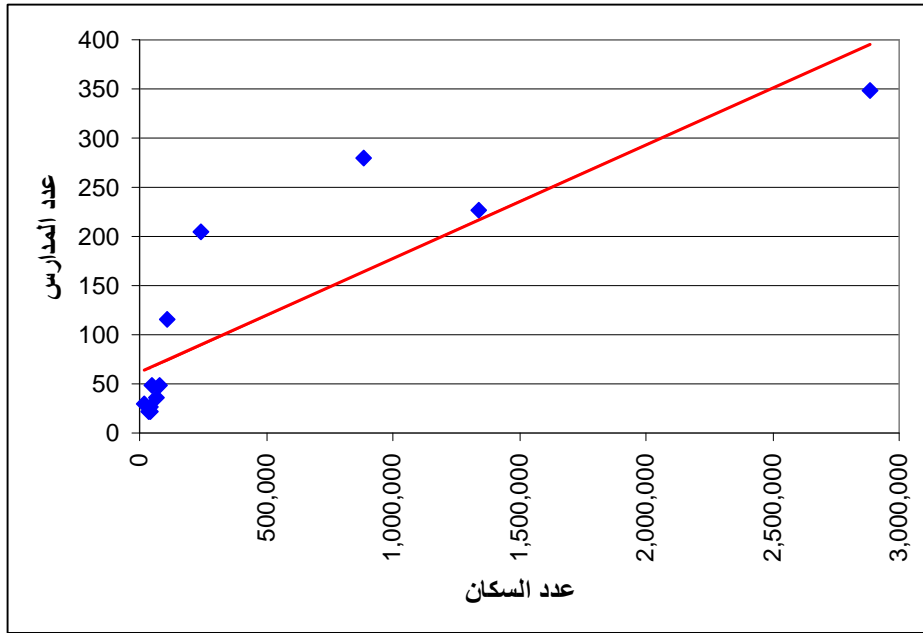
شكل (٢-٦) خط الانحدار
