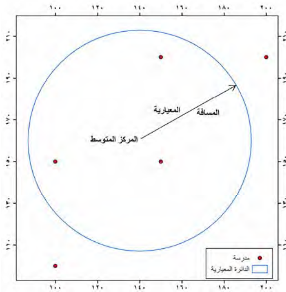
شكل (٣-٣) المسافة و الدائرة المعيارية
