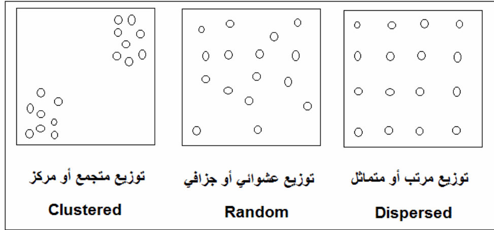
شكل (٥-٣) أنواع أو أنماط التوزيعات
