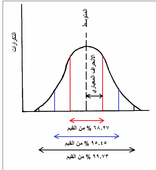
شكل (٢-١) منحني التوزيع الطبيعي
