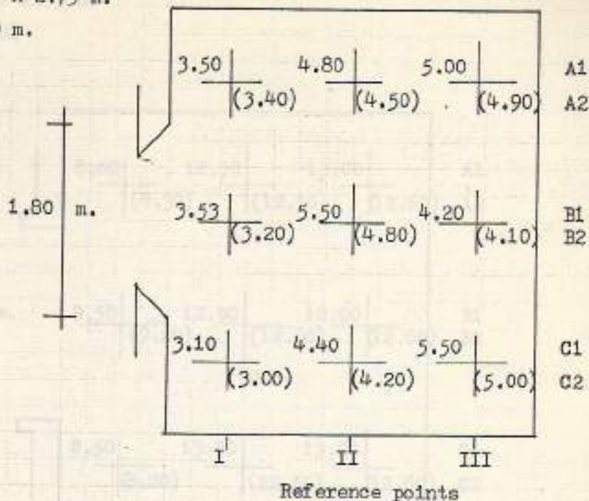
Plan 1:50
