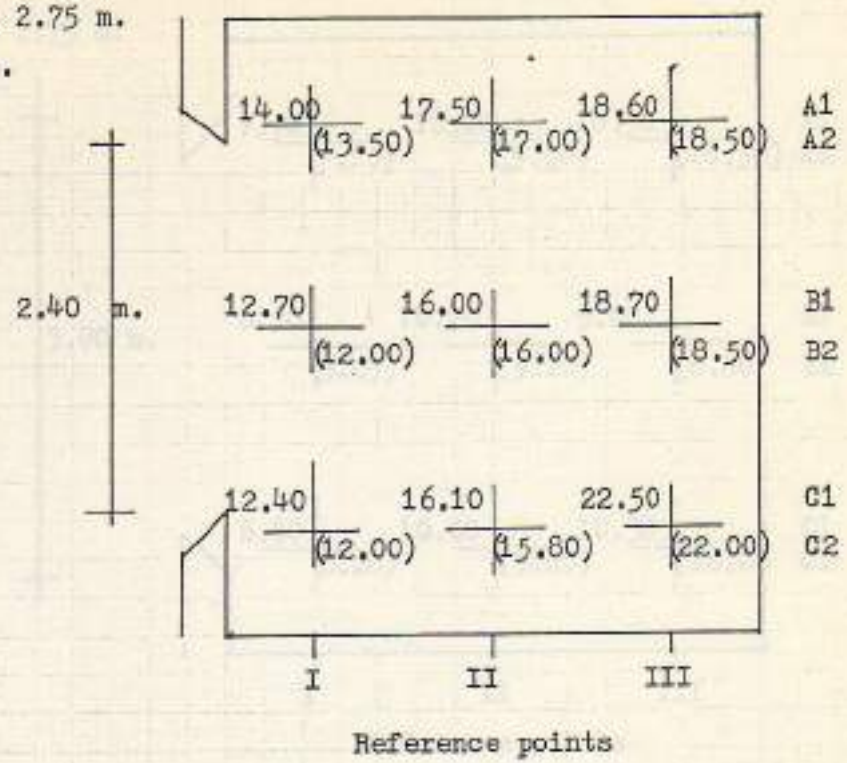
Plan 1:50
