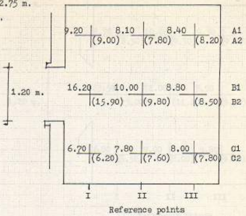
Plan 1:50
