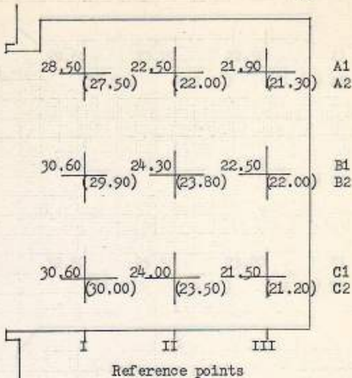
Plan 1:50
