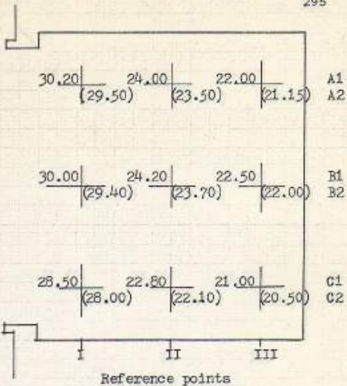
Plan 1:50
