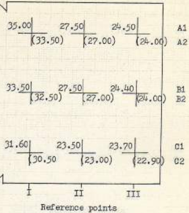
Plan 1:50
