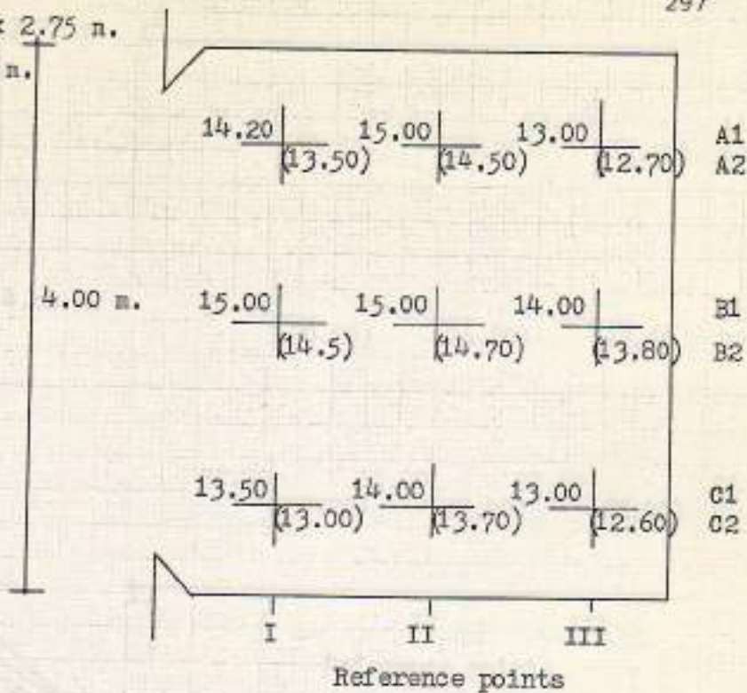
Plan 1:50
