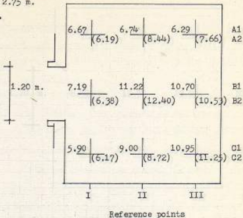
Plan 1:50
