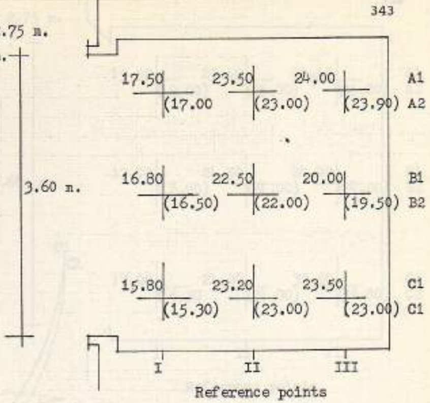
Plan 1:50
