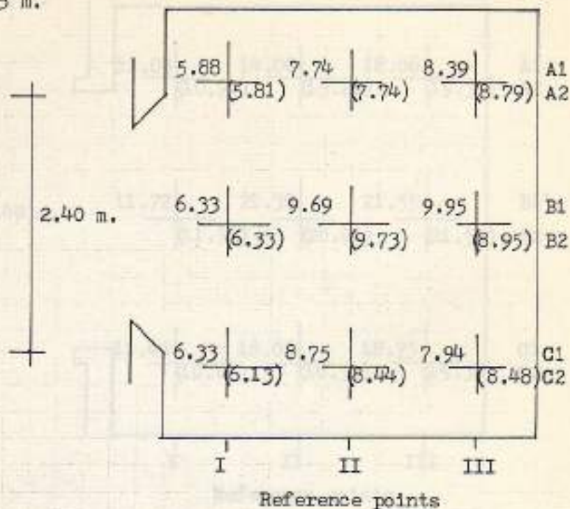
Plan 1.:50
