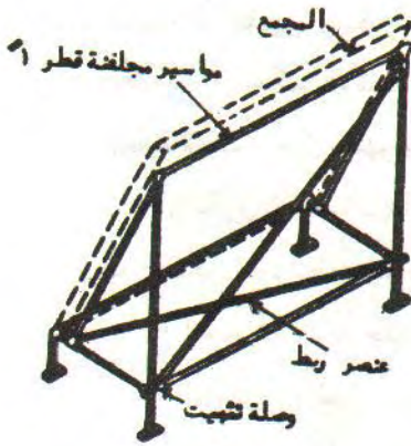
١ - السطح الجمع للأشعة مثبت على هيكل من المؤاسير المجلفنة
