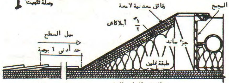
ب - السطح الجمع للأشعة ملتصق بالسطح
