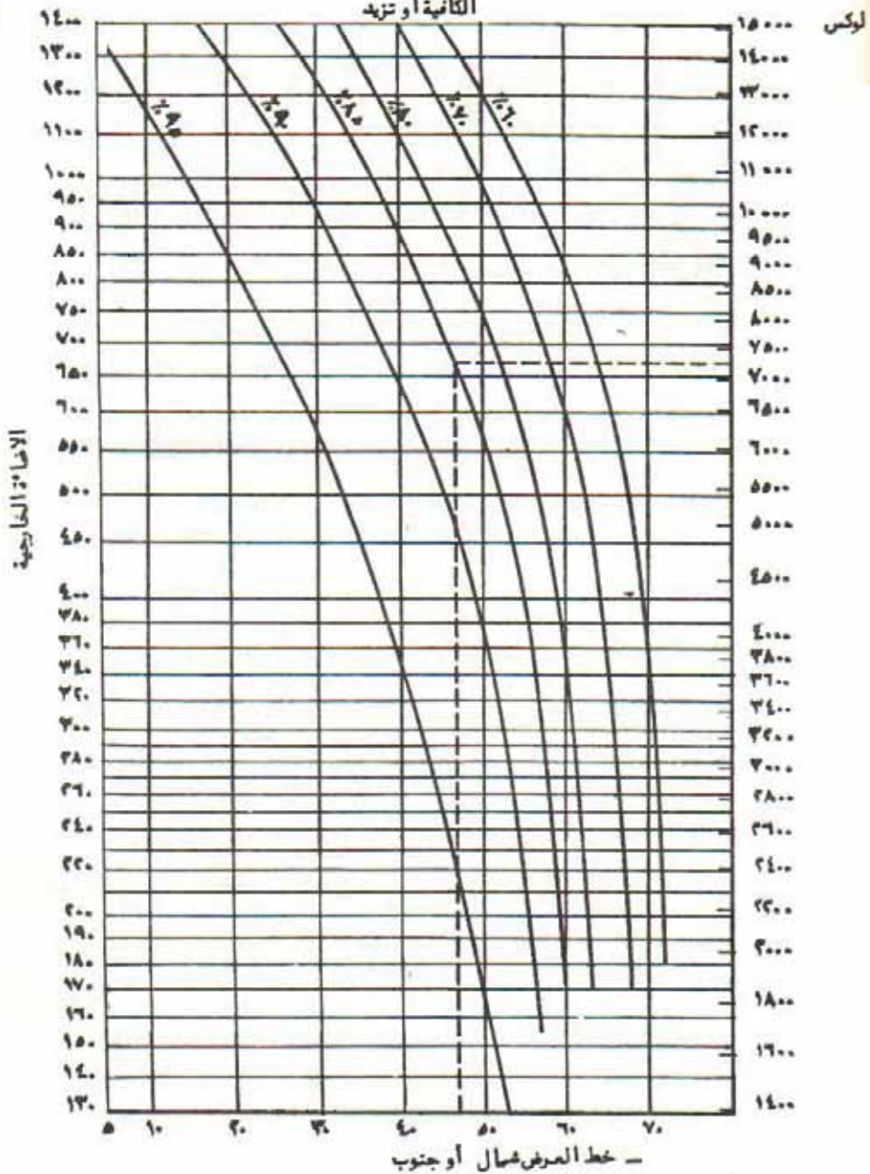
شكل ١٠٤ : العلاقة بين الحد الأدنى للإضاءة الخارجية وخط العرض والنسبة المثوية للساعات التي تتوفر فيها شدة الإضاءة الكافية
