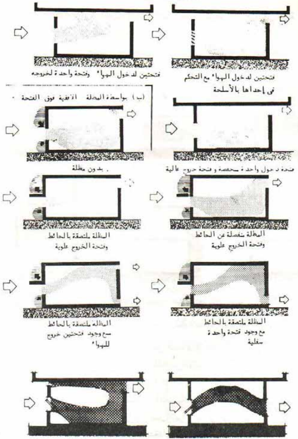
(ج) توجيه الهواء* لأعلى ولأسفل باستخدام الشباك السحوري شكل ٦٥ : توجيه الهواء داخل الغرفة
