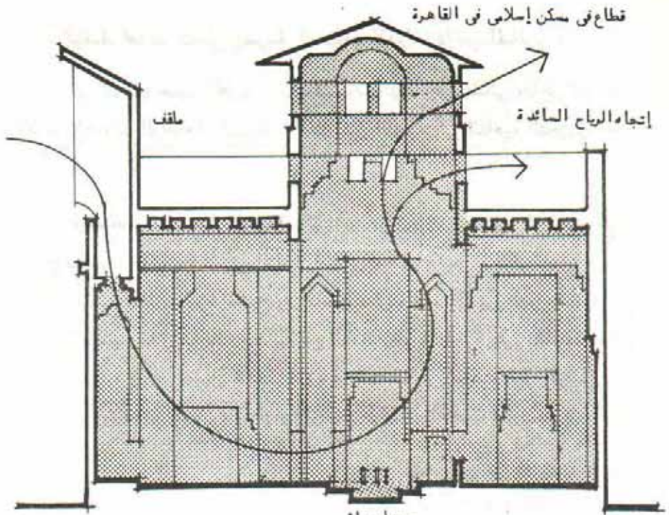
شكل ٧٨ : سحب الهواء الساخن لأعلى ثم للخارج بواسطة المدخنة ويدخل الهواء المنعش سواء من فتحة شباك في جدار الخارجى أو من ملفف
