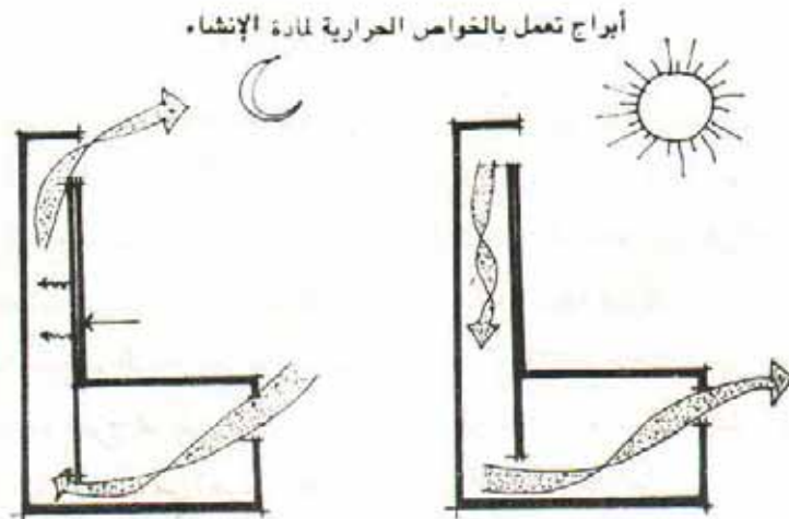
شكل ٦٩ : التقسيم الأساسي لأبراج الرياح
