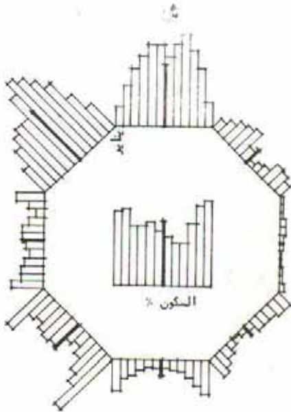
شكل ٥٦ (ب) : وردة الرياح لمدينة العريش
