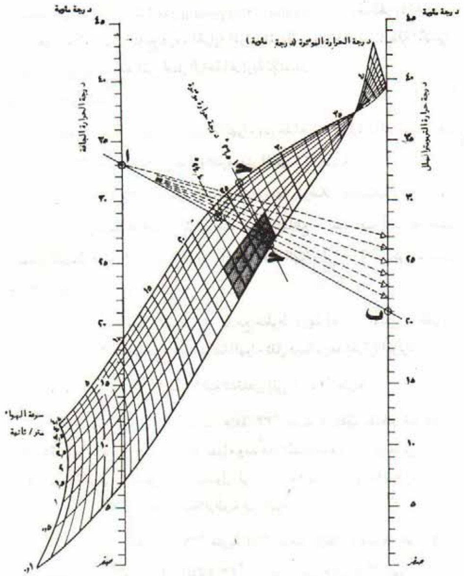
شكل ١١٢ : مقياس درجة الحرارة المؤثرة لأشخاص يرتدون ١ كلو ويقومون بأعمال مكتبية معتادة
