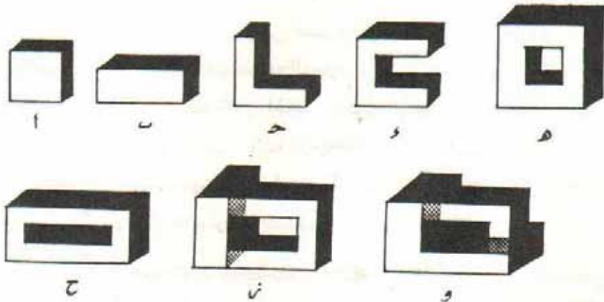
شكل ٢٤ : تأثير شكل المبنى على كمية الظلال الساقطة . من الواضح أن أكبر كمية ظلال تكون في المبنى متعدد الأدوار ذي الحوش الداخلي
