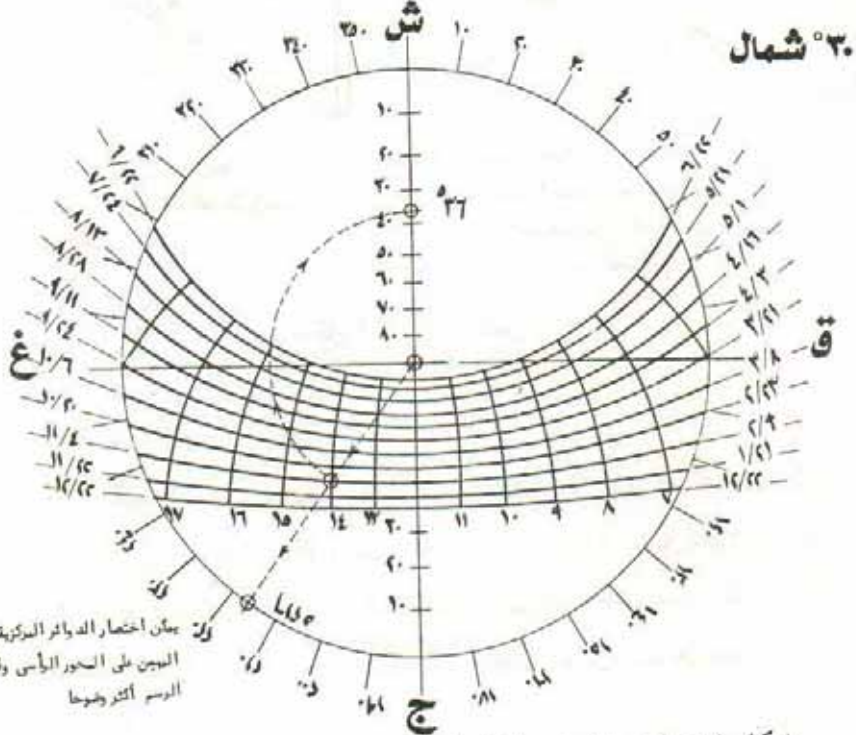
شكل ١١ : استخدام خريطة المسار الشمسي في تعيين زوايا سقوط الشمس
