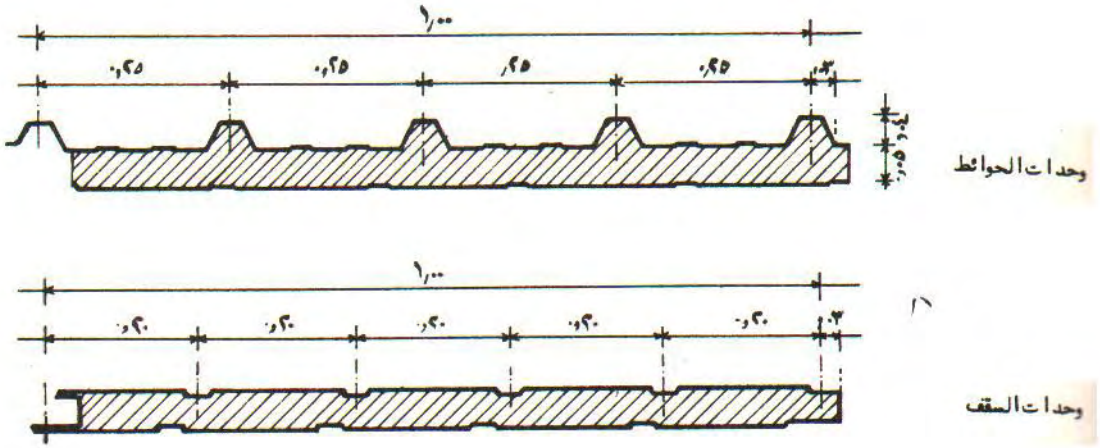
شكل ٤٢ : الألواح المعزولة Sandwich Panel
