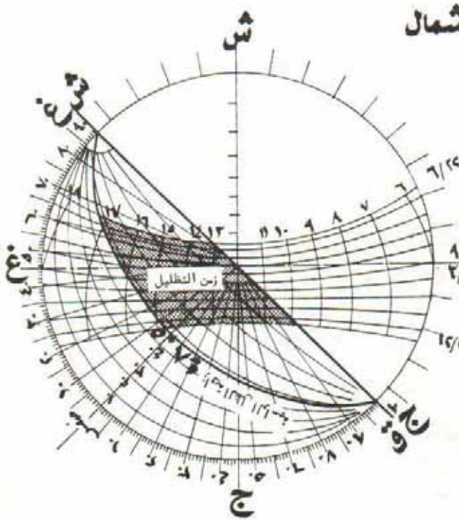
الظل الناتج عن الكاسر الأفقي أ
