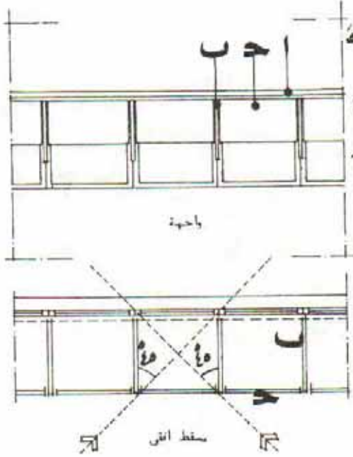
شكل ٣٠ : طريقة عمل قناع الإطلال لواجهة معلومة
