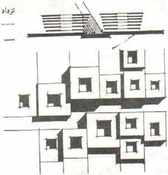
شكل ١٥ : تأثير شكل تجميع المباني فى كمية الظلال الساقطة
