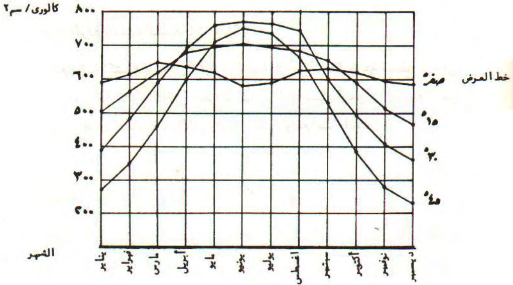
شكل ٣٦ (أ) كمية الإشعاع الشمسى اليومية الساقطة
