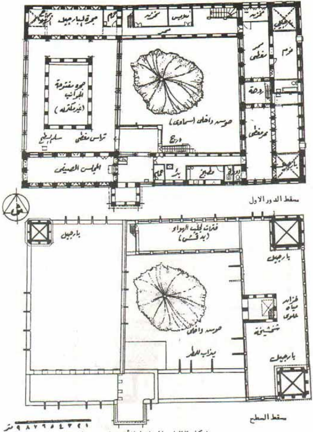
شكل ١٢٢ : المساقط الأفقية لوحدة سكنية
