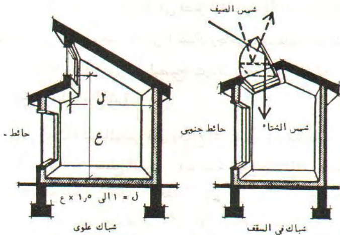
شكل ٤٩ : أشكال الفتحات العلوية المُستقبلة لأشعة الشمس
