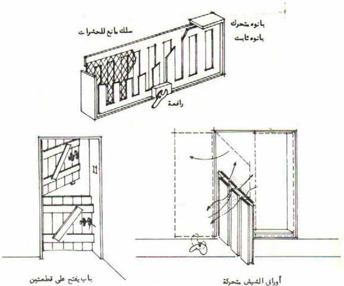
شكل ١٣١ : تفاصيل تساعد على التحكم فى التهوية
