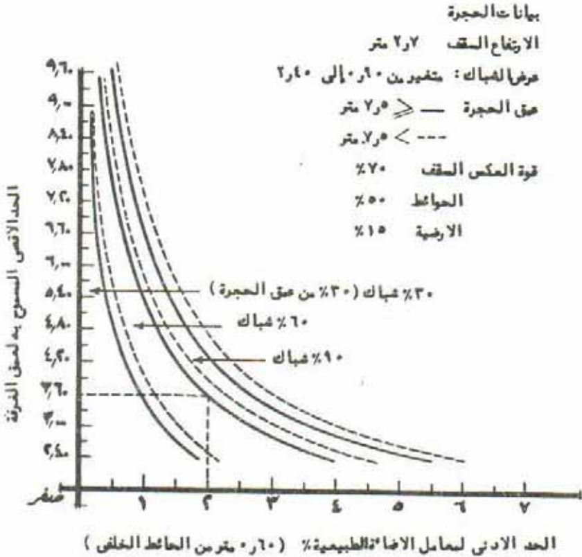
شكل ١٠٢ : منحني CIE
