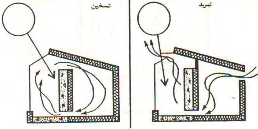
شكل ٤٧ : طريقة الفراغ الشمسي
