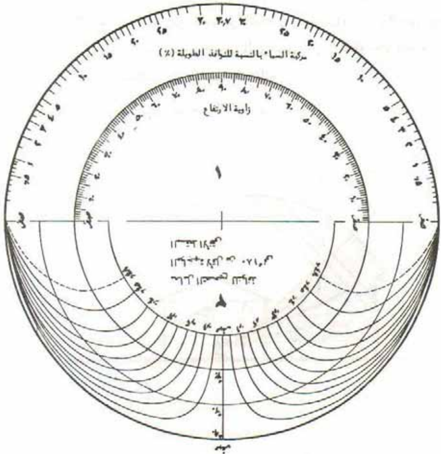
شكل ٩٤ : منقطة الإضاءة الطبيعية
