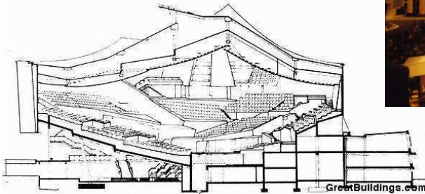
شكل ( ١ - ٤١ ) قطاع رأسي يمر بالقاعة
