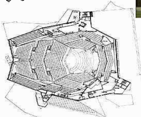
شكل ( ١ - ٣٩ ) مسقط أفقي للقاعة
