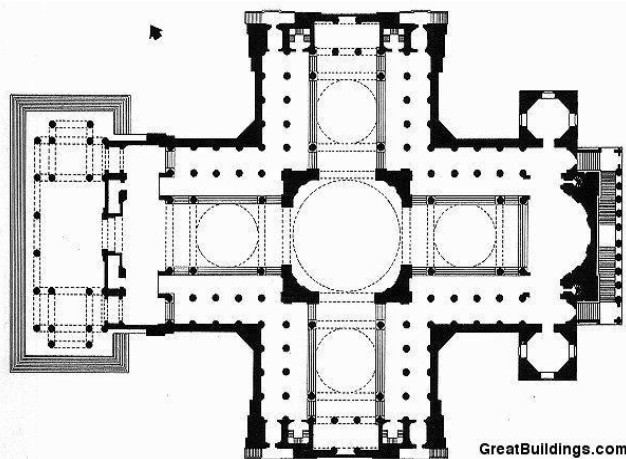
شكل ( ١ - ١١ ) المسقط الأفقي لمبنى البانثيون ( ٣ )
