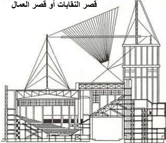
شكل (١ - ٢٥) قطاع قصر النقابات أو قصر العمال
